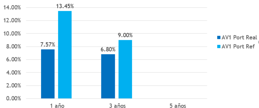
SURA AV1 VS Portafolio de Referencia
